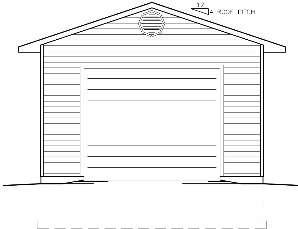
END ELEVATION
